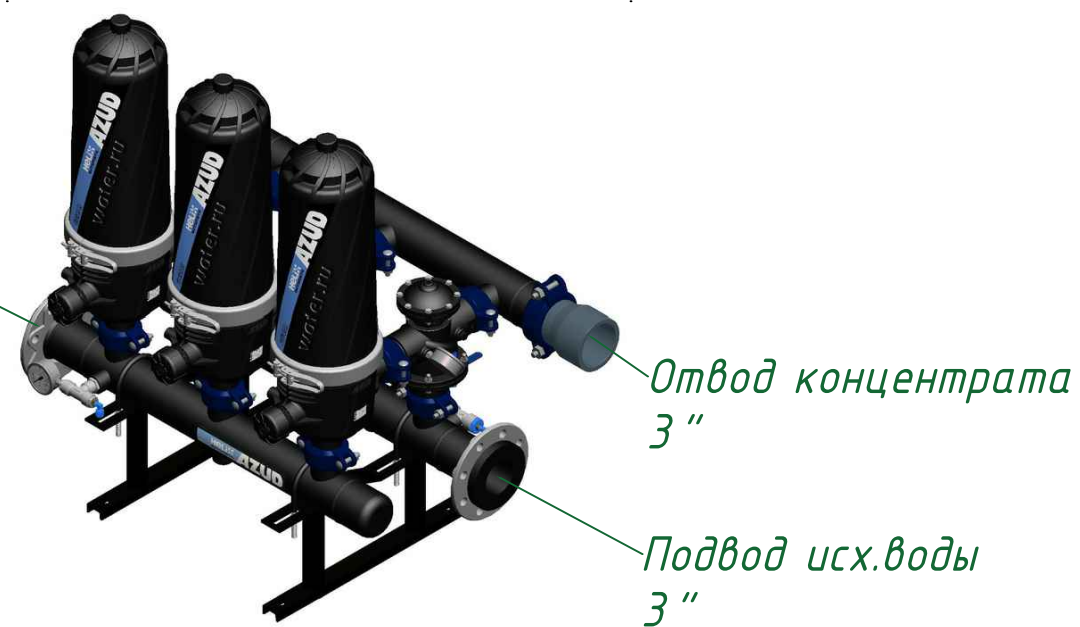
Изометрия
