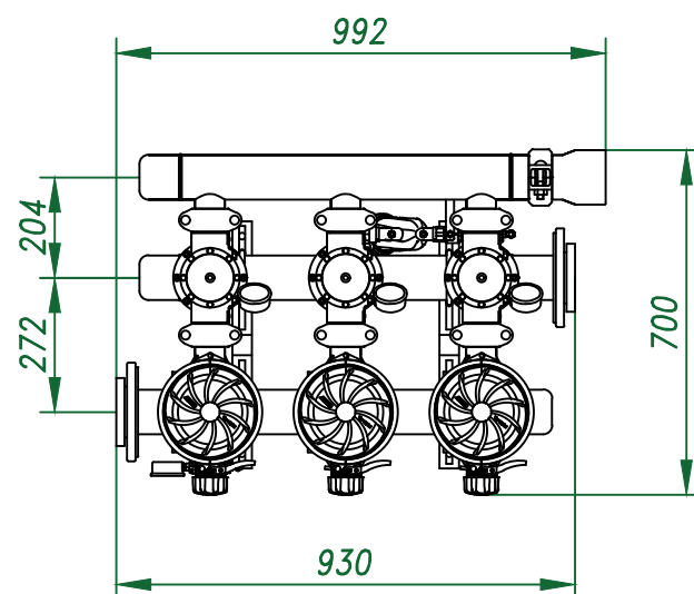
Вид сверху
