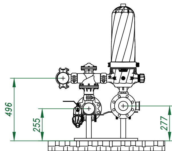
Вид слева
